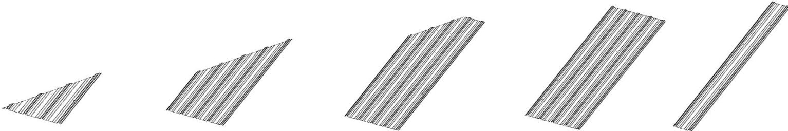
A4M01359-1 29GA STEEL SHEETING (x1) A4M01358-1 29GA STEEL SHEETING (x1) A4M01357-1 29GA STEEL SHEETING (x1) A4M01240 29GA STEEL SHEETING (x1) A4M01899 29GA STEEL SHEETING (x1)
