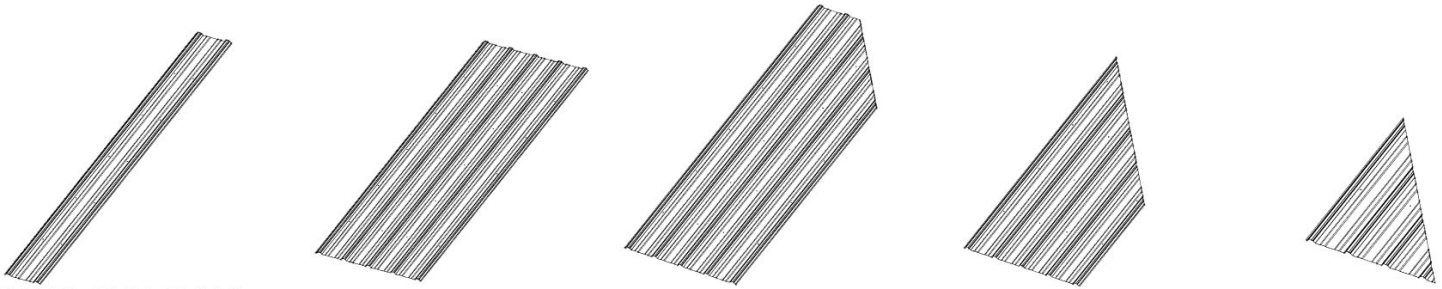
A4M01899 29GA STEEL SHEETING (x1) A4M01240 29GA STEEL SHEETING (x1) A4M01354-1 29GA STEEL SHEETING (x1) A4M01355-1 29GA STEEL SHEETING (x1) A4M01356-1 29GA STEEL SHEETING (x1)
